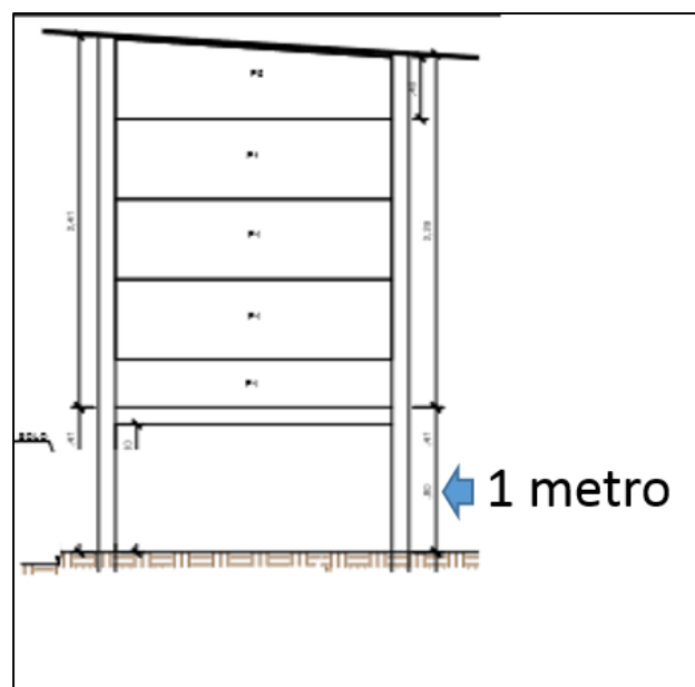
Figura 2: Desenho técnico de uma instalação sanitária domiciliar desenhada para ambiente de várzea.
