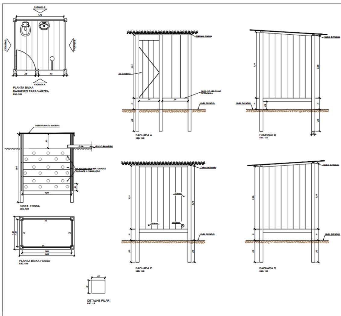
Figura 3: Instalação Sanitária Domiciliar de madeira adequada para ambiente de Várzea
