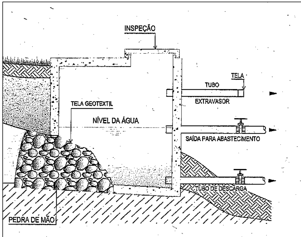
Figura 3: Modelo esquemático da caixa de tomada para captação da água de nascente de encosta.
