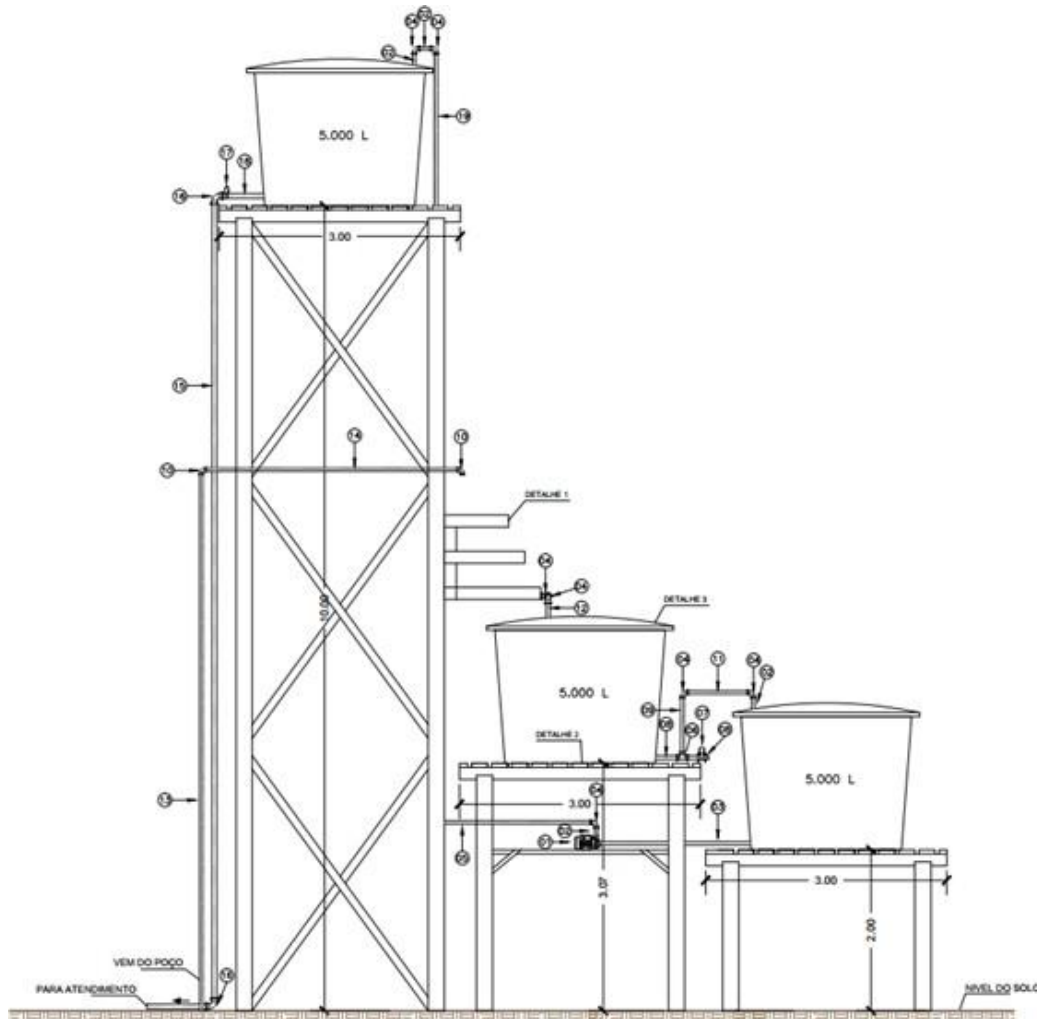
Figura 10: Desenho esquemático do sistema de abastecimento complementar.
