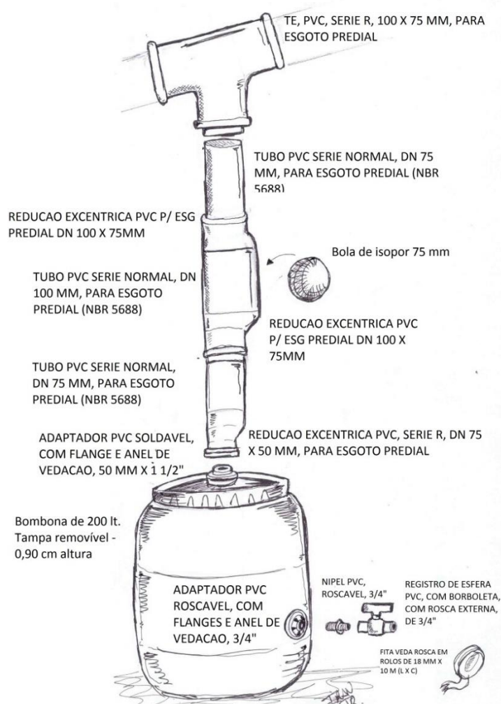
Figura 18: Modelo do dispositivo de descarte automático
