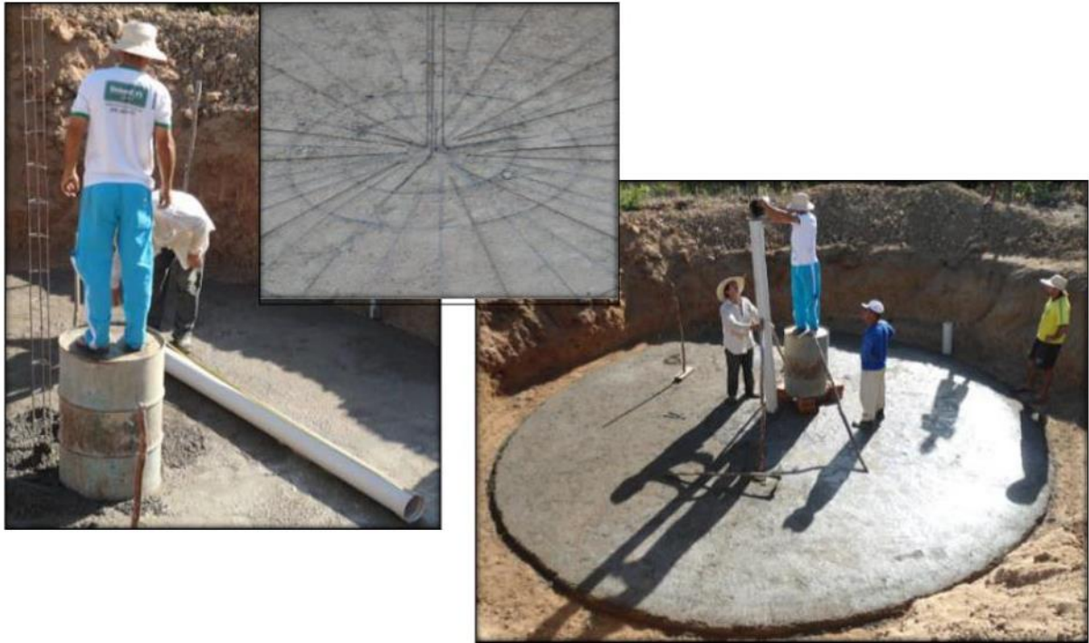
Figura 10: Construção da Coluna Central
