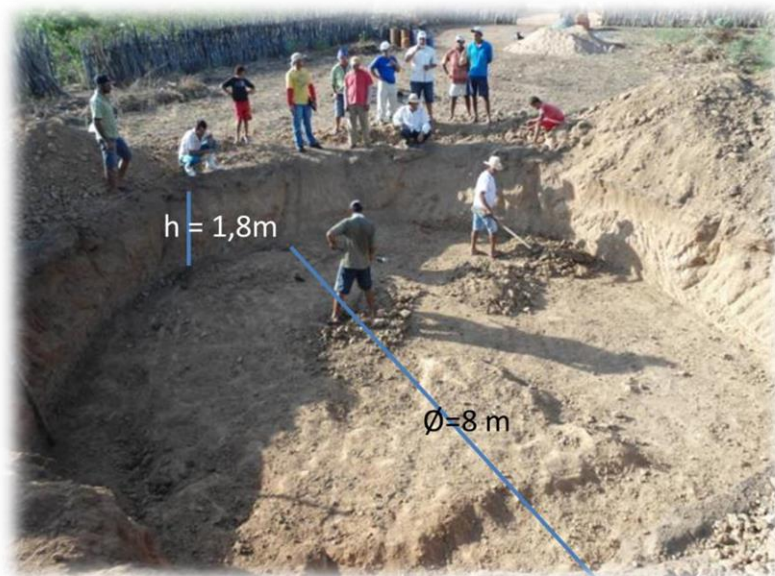
Figura 3: Escavação - acabamento manual do fundo da escavação
