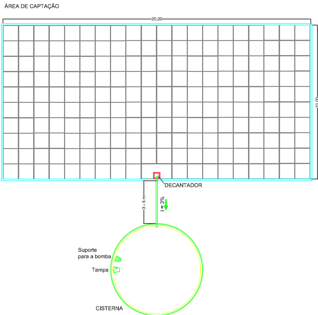
Figura 1 – Desenho esquemático do calçadão
